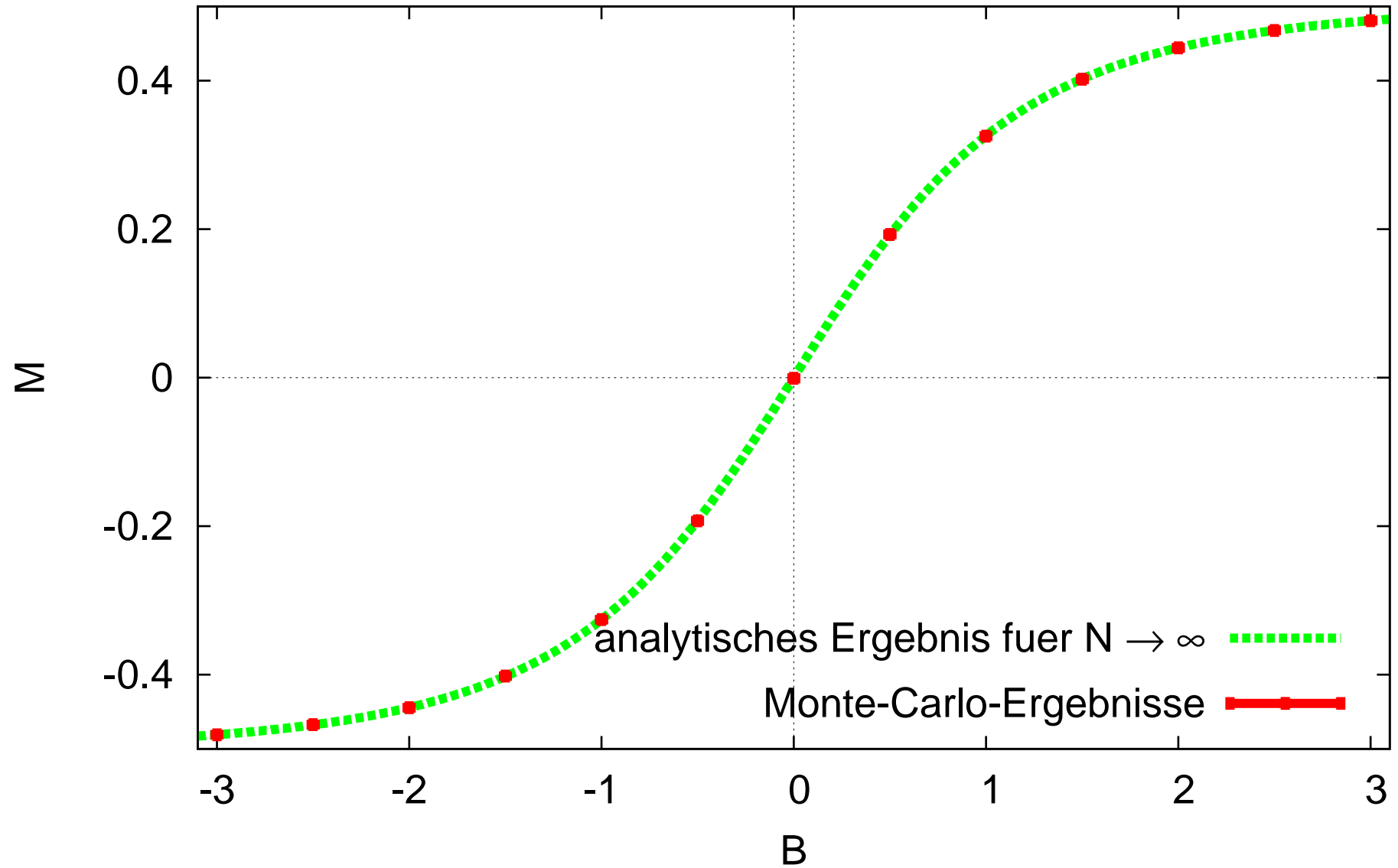
M als Funktion von B ( \beta = 1.0 , N = 1000 , \lambda = 1.0 )
