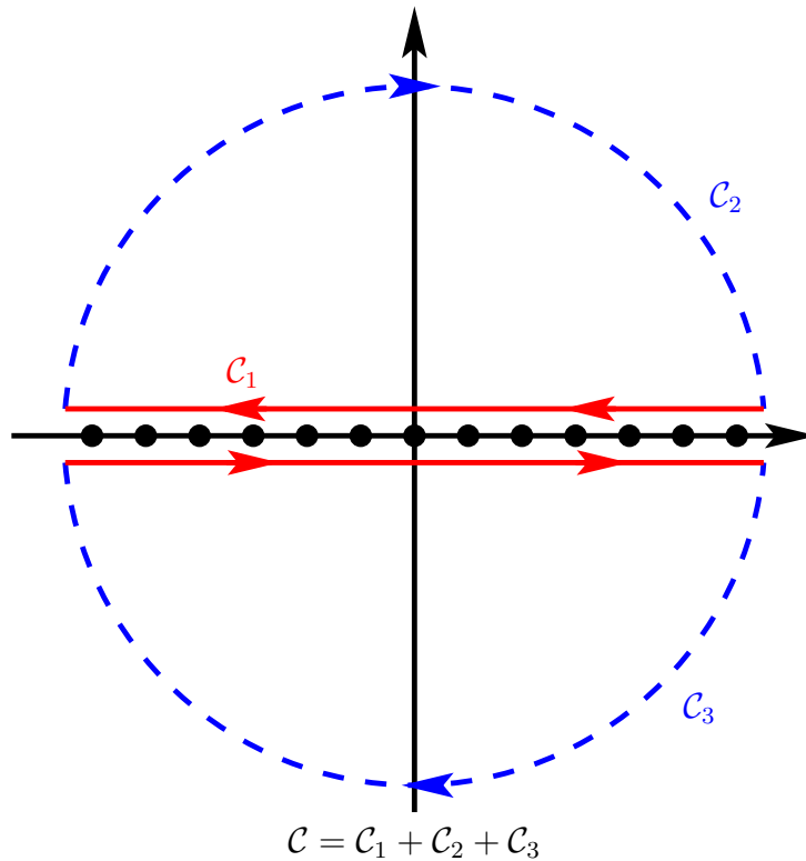
Abbildung 7.1: Kontur zur Integration der Funktion (7.5.27).
