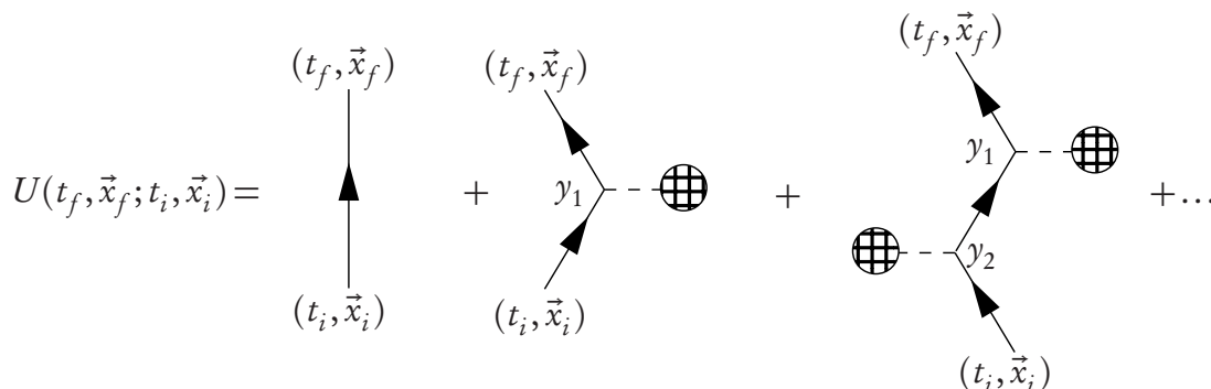
Abbildung 7.2: Diagrammatische Darstellung der Born-Reihe.
