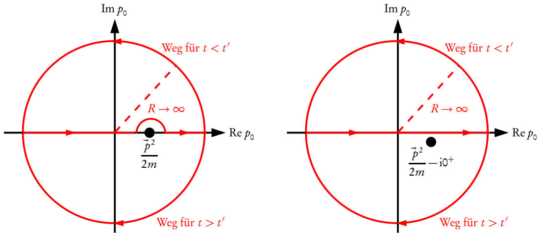
Abbildung 2.1: Links: Integrationskontur für das Integral (2.14.15) für den retardierten Propagator . Rechts: Alternative Formulierung durch Verschieben des Pols in die untere Halbebene (cf. (2.14.18) und Beibehaltung des ursprünglichen reellen Integrationsweges.
