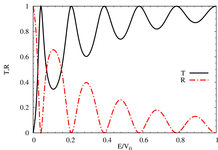
Abbildung 3.5: Transmissions- und Reflexionskoeffizienten beim Potentialtopf.
