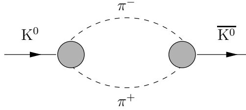
Abbildung 1: Die Kaonenooszillation in effektiven Modellen der schwachen Wechselwirkungen von Hadronen: Das Zweipionen-Austauschdiagramm führt zu einer „spontanen“ Umwandlung eines Kaons in ein Antikaon und zurück (man kann die Pfeile auch einfach umkehren).
